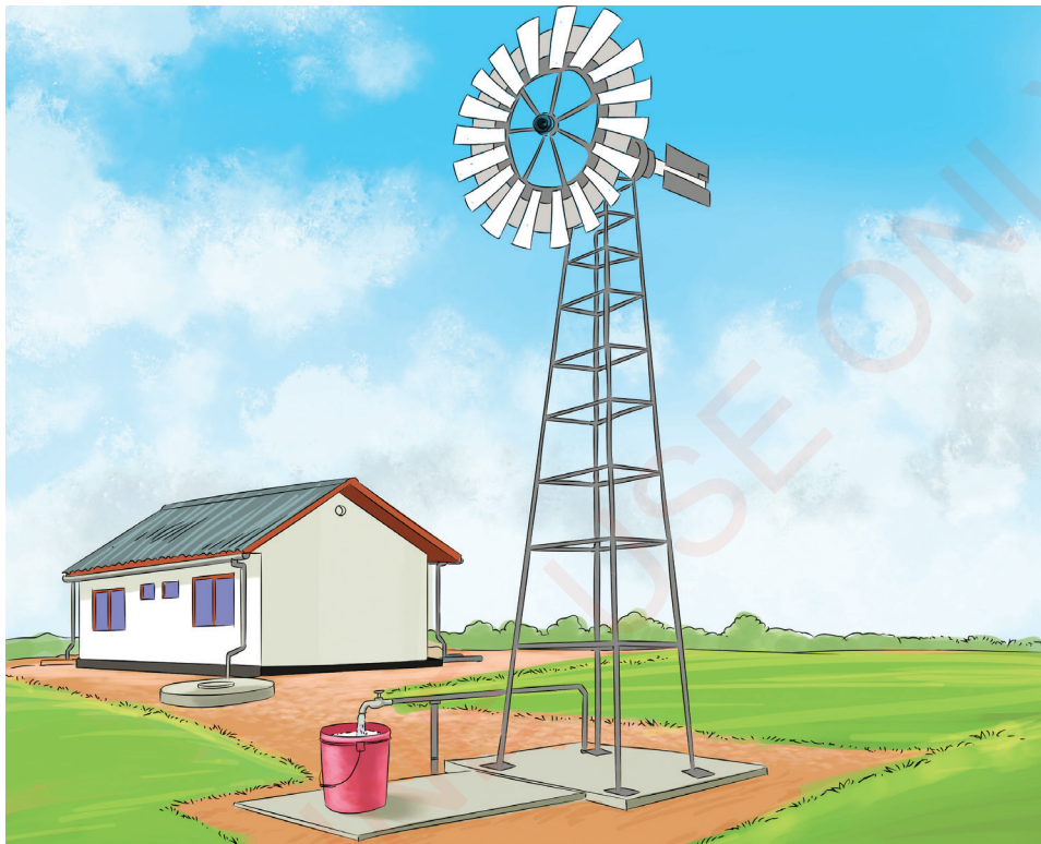
Kielelezo namba 1: Kinuupepo kikivuta maji kutoka ardhini
